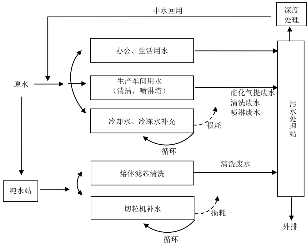
图 B.6 聚酯生产中用水、排水与水的循环使用示例图
